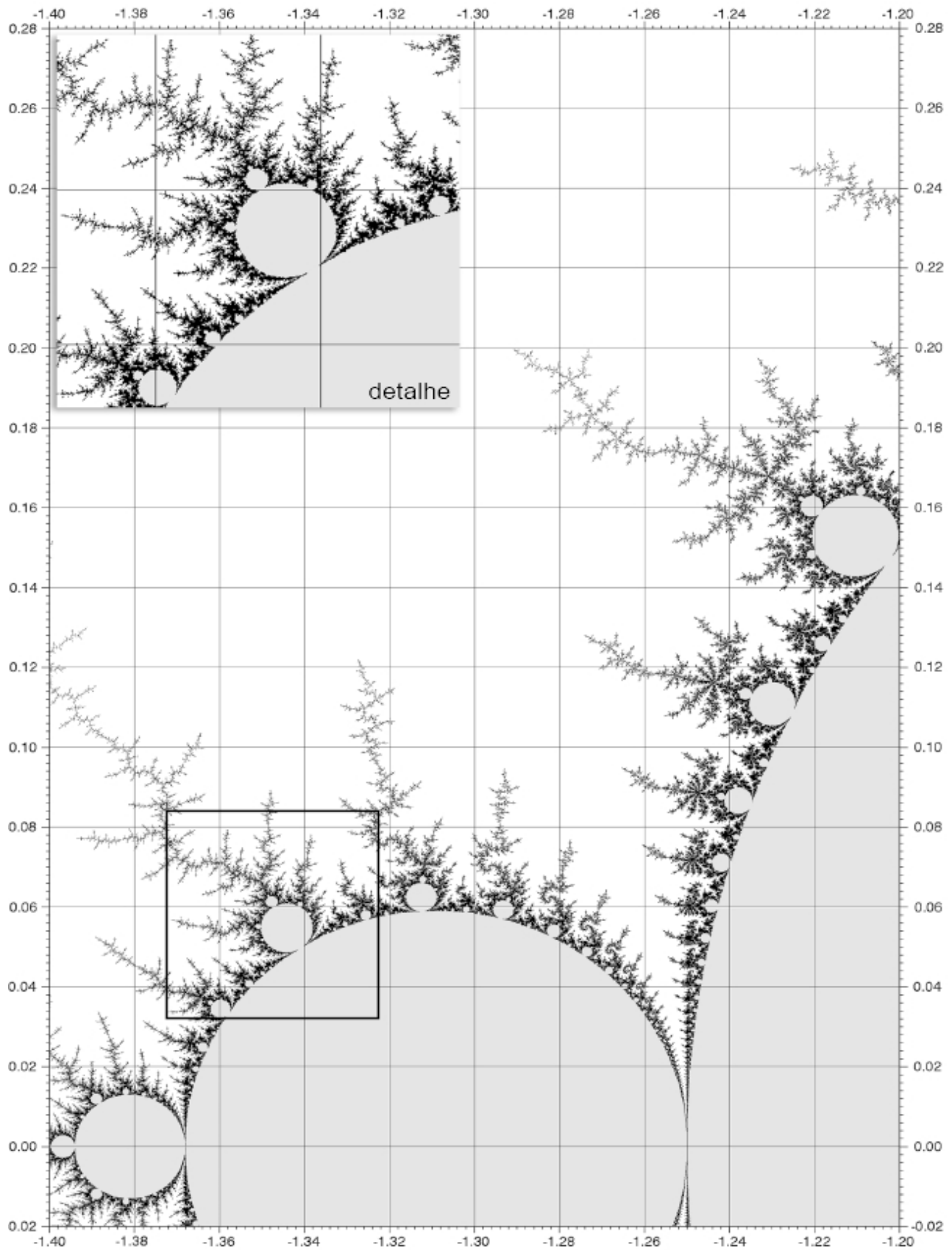
O conjunto de Mandelbrot
