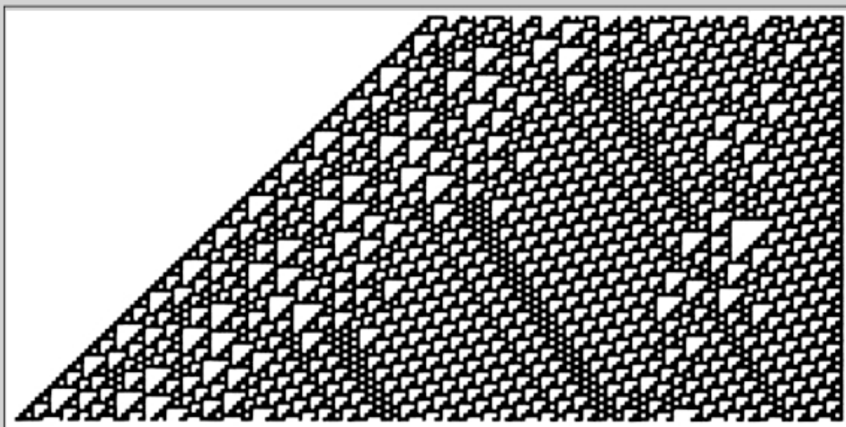
Porção da imagem gerada pela Regra 110
